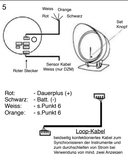
Rückansicht
