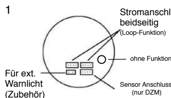
Rückansicht
