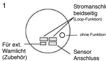
Rückansicht
