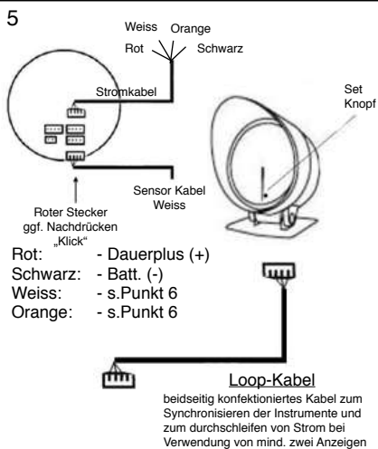
Rückansicht
