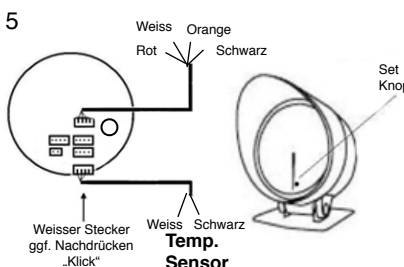
Rückansicht
